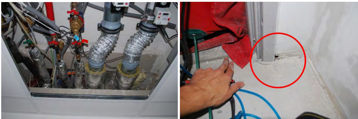
Abbildung 36: Fehlendes Weichschott beim Schachtabschluss (links) und Lufttritt im Bereich der Türzarge (rechts) [Quelle: Ingenieurbüro Filos]
