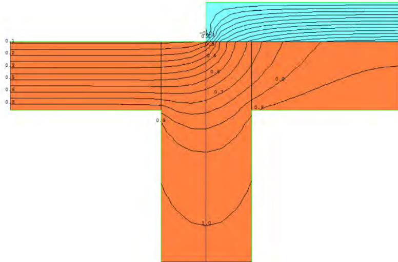
Abbildung 35: Isothermen-Darstellung. Wärmebrücke Außenwand – Feuermauer [Quelle: Schöberl & Pöll GmbH]
