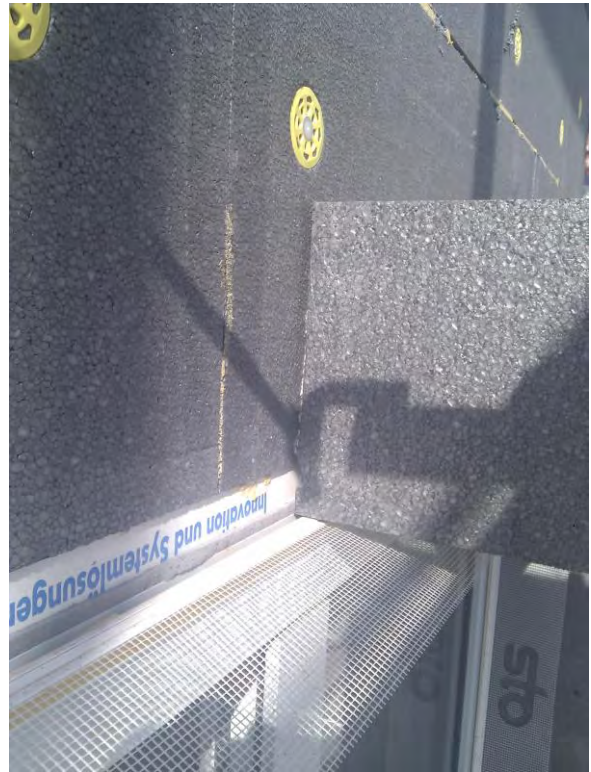
Abbildung 28: Positionierung der Fenster in der Dämmebene (links) und Überdämmung des Fensterstockes (rechts) [Quelle: Schöberl & Pöll GmbH]
