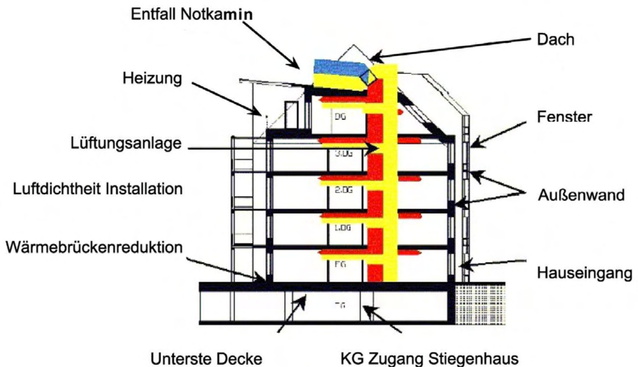
Abbildung 3: Komponenten für die Passivhaus-Sanierung [SCH09]
