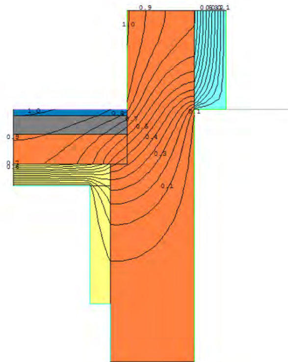
Abbildung 31: Isothermen-Darstellung. Wärmebrücke tragende Außenwand – Kellerdecke (ohne Kragendämmung außen und mit Kragendämmung innen) [Quelle: Schöberl & Pöll GmbH]
