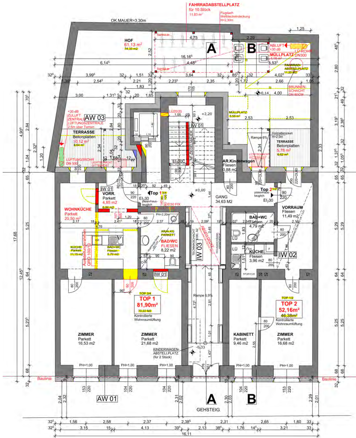
Abbildung 16: Grundriss Erdgeschoss [Quelle: Ageres Baumanagement]
