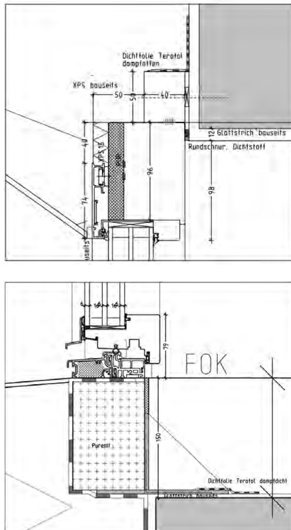
Abbildung 25: Vertikalschnitt Fensteranschluss beim Projekt Eberlgasse [PSP Holz GmbH]
