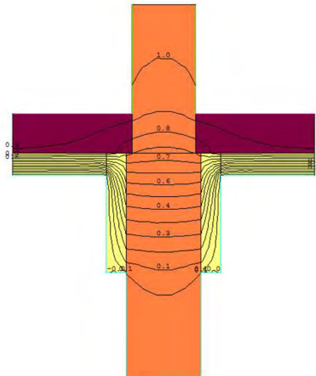
Abbildung 34: Isothermen-Darstellung. Wärmebrücke tragende Innenwand – Kellerdecke [Quelle: Schöberl & Pöll GmbH]
