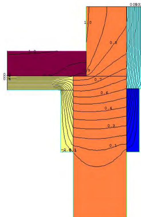
Abbildung 32: Isothermen-Darstellung. Wärmebrücke tragende Außenwand – Kellerdecke (mit Kragendämmung außen und innen) [Quelle: Schöberl & Pöll GmbH]
