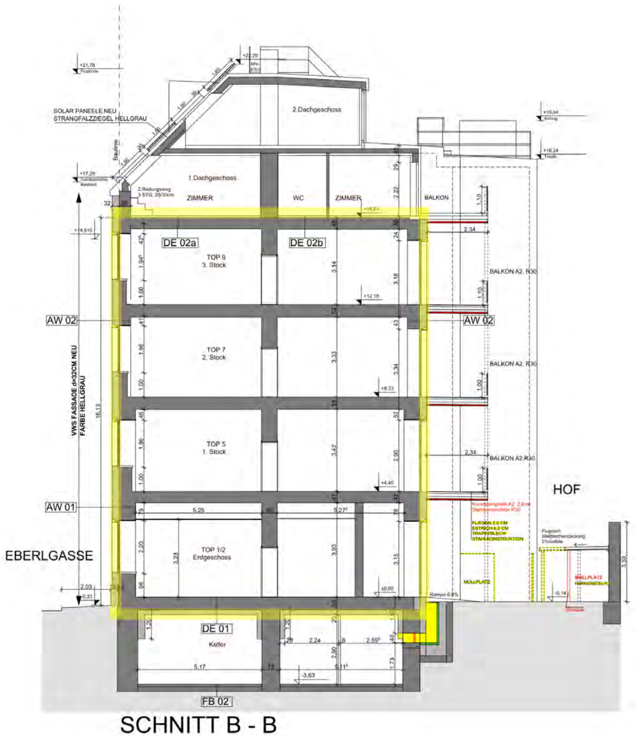
Abbildung 15: Gebäudeschnitt mit eingezeichnetem Verlauf der thermischen Gebäudehülle [Quelle: Ageres Baumanagement, bearbeitet von: Schöberl & Pöll GmbH]
