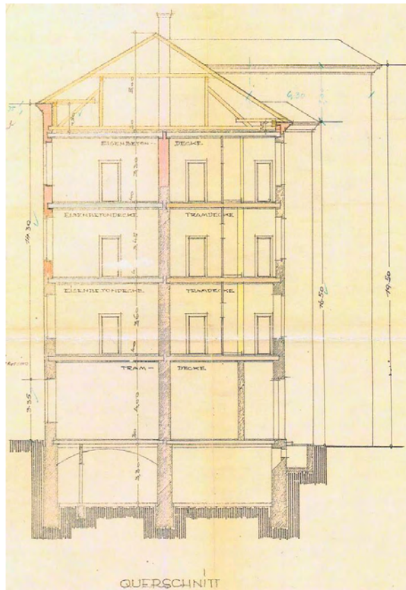
Abbildung 13: Wiederaufbauplan 1948 - Bestandsschnitt Eberlgasse [Quelle: Andreas Kronberger]
