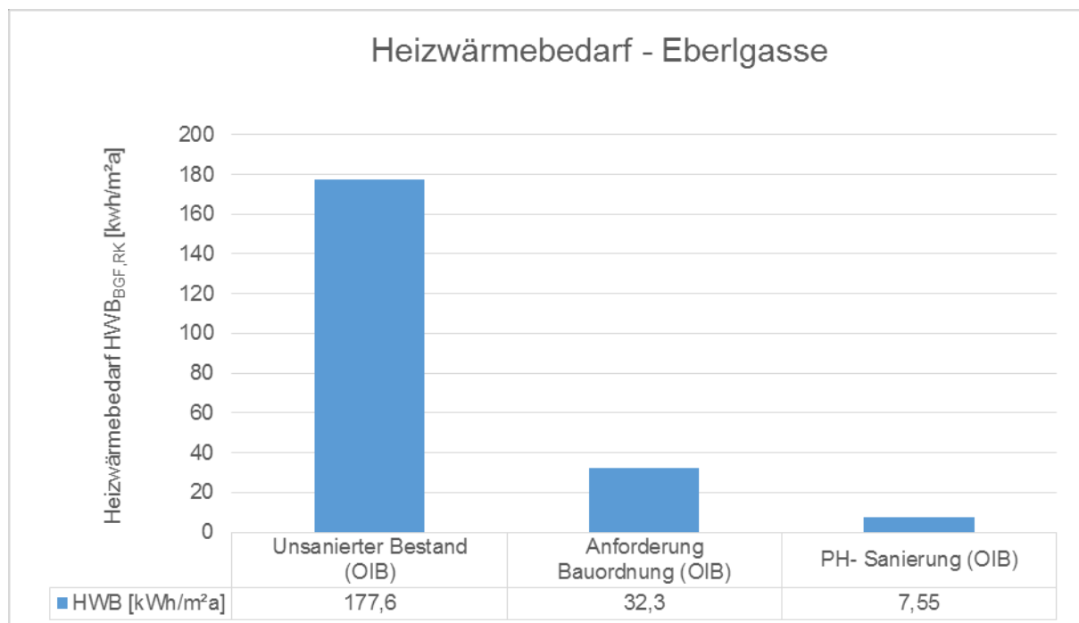
Abbildung 51: Vergleich Heizwärmebedarf [kWh/m BGF *a] unsaniertes Bestand, Anforderung gemäß OIB Richtlinien 6 (Ausgabe 2011) und saniertes Passivhaus Eberlgasse [Quelle: Schöberl & Pöll GmbH]
