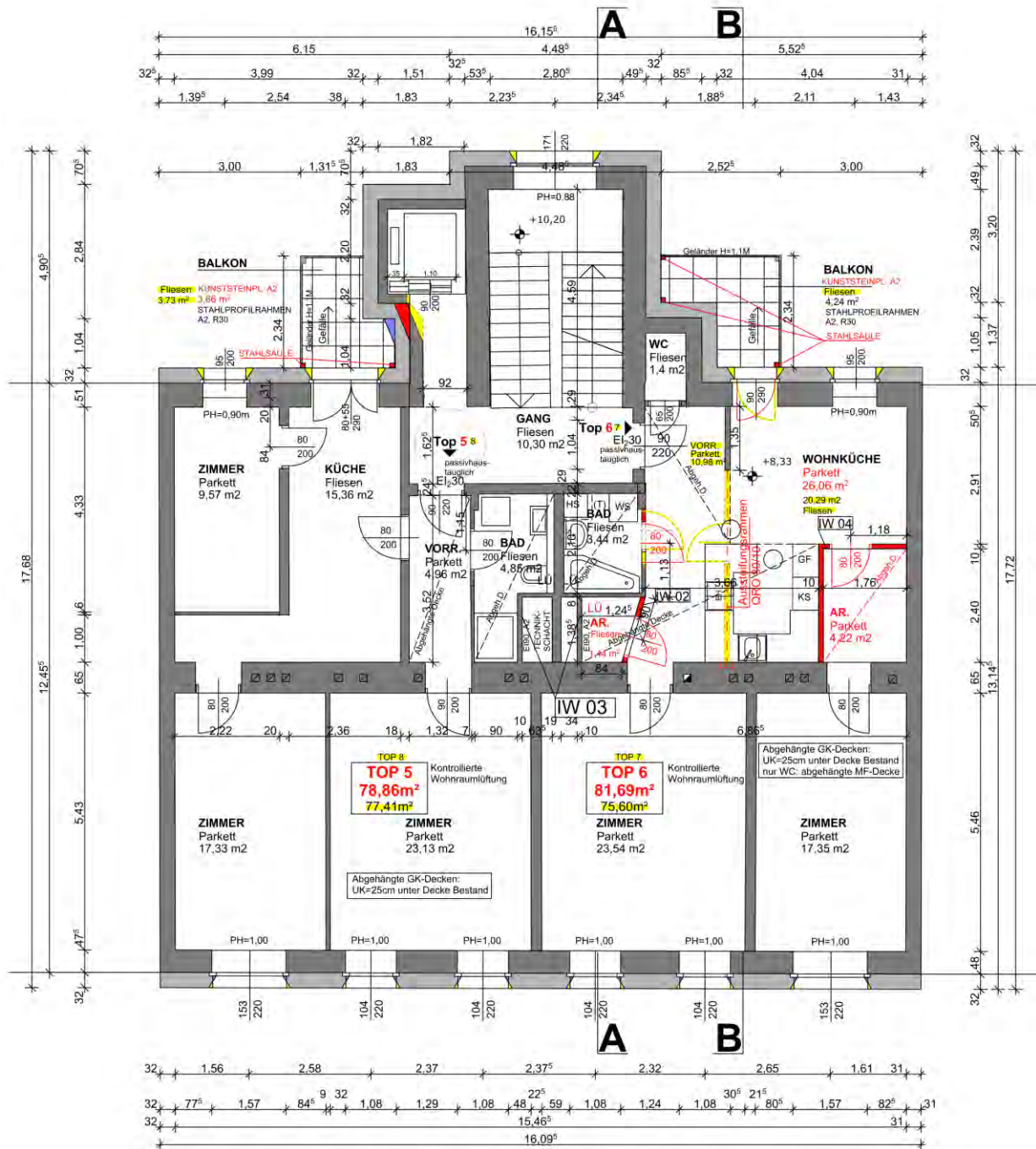
Abbildung 17: Grundriss 2.Obergeschoss [Quelle: Ageres Baumanagement]
