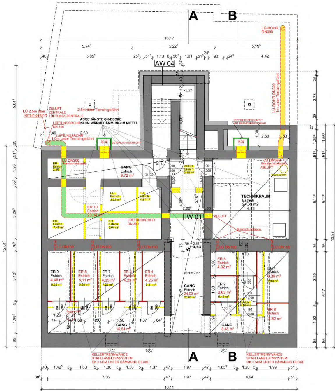
Abbildung 38: Grundriss Kellergeschoß mit Lage der haustechnischen Komponenten [Quelle: Ageres Baumanagement]
